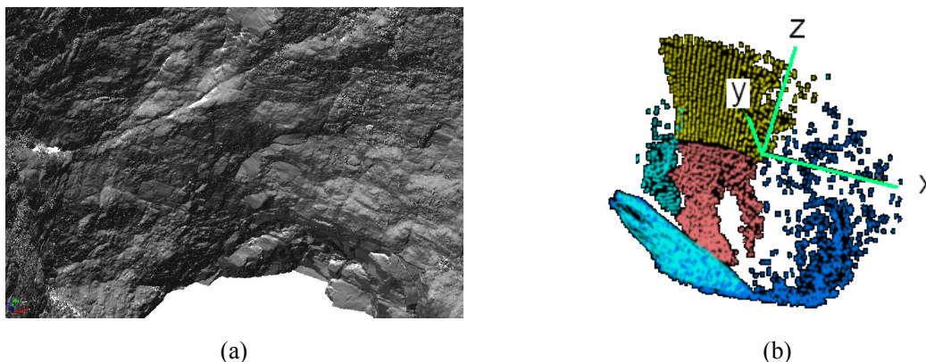
Slika 1.14 Oblak točkaca mjereno TLS uređajem na a) primjeru Crvenog jezera te b) mjereno fotogrametrijskom metodom na primjeru Modrog jezera kod Imotskog
