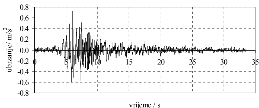
Crtež 4.14 Vremenski zapis ubrzanja za vrijeme potresa u Petrovcu 1979.
