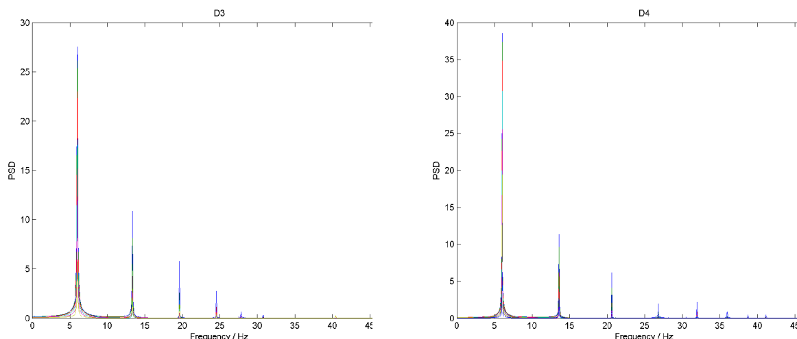
Slika 8. 19 Spektri odgovora
