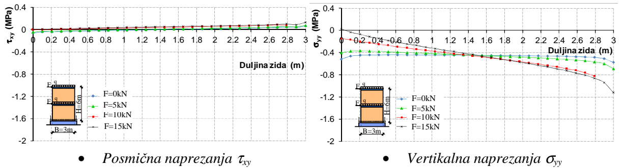
(i) Zid URM 1
