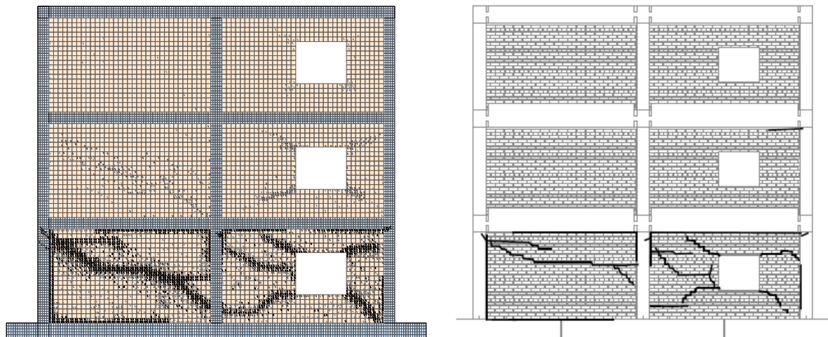
(i) Stanje pukotina - numerički model prikazan u Poglavlju 2
