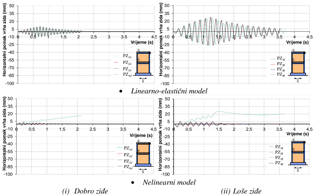
Slika 5.124. Horizontalni pomak vrha zidanih zidova bez otvora
