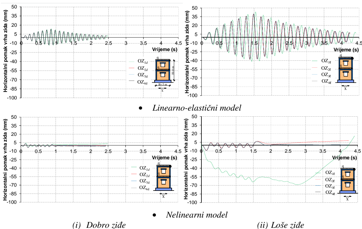
Slika 5.125. Horizontalni pomak vrha zidanih zidova s otvorima
