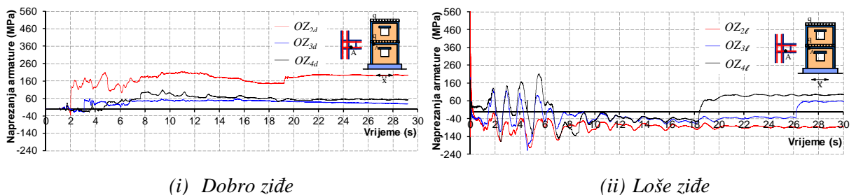
Slika 5.113. Utjecaj promjera uzdužnih šipki horizontalnog serklaža na naprezanje armature u točki A donjeg horizontalnog serklaža zidanih zidova s otvorima
