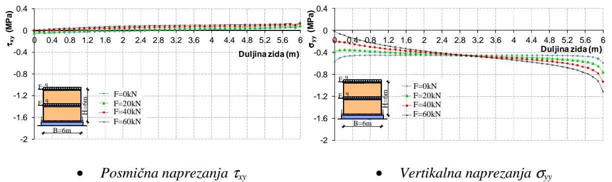
(ii) Zid URM 2
