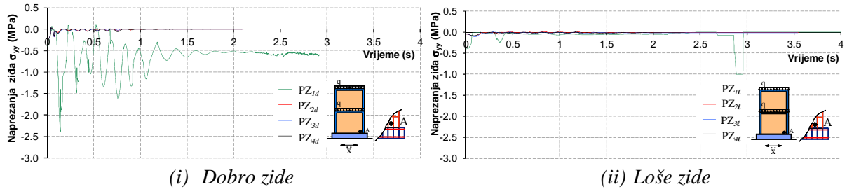
Slika 5.41. Vertikalno naprezanje u žiđu u točki A pri dnu zidanih zidova bez otvora
