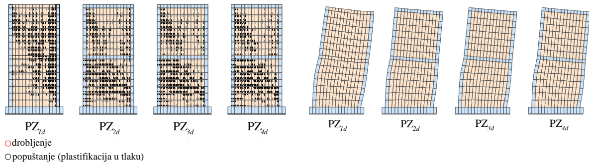
(i) Pukotine (ii) Pomaci (uvećano 100 puta)
