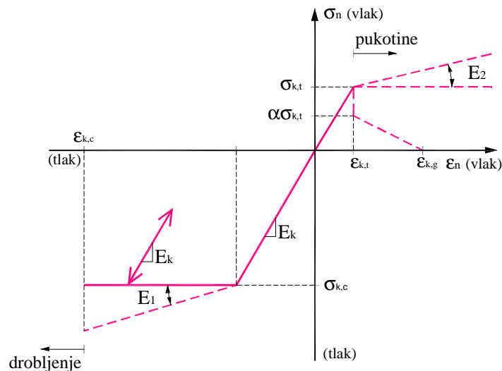
Slika 2.35. Modeliranje prijenosa normalnog naprezanja 2D dodirnog elementa
