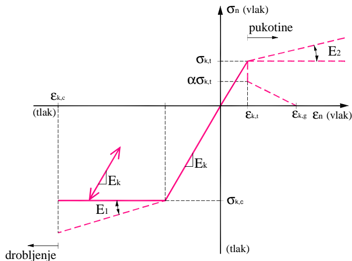
Slika 2.35. Modeliranje prijenosa normalnog napreznja 2D dodirnog elementa
