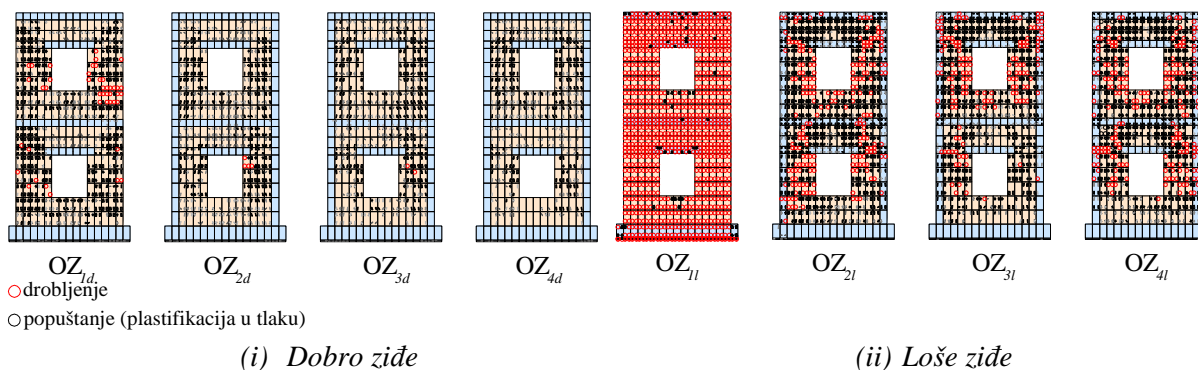
Slika 5.48. Stanje pukotina u zidanim zidovima s otvorima nakon prestanka djelovanja harmonijske pobude
