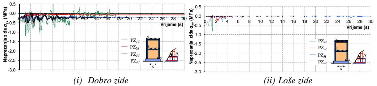
Slika 5.79. Vertikalno naprezanje u zidu u točki A pri dnu zidanih zidova bez otvora
