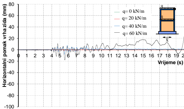
Slika 5.18. Horizontalni pomak vrha narmiranih zidanih zidova s otvorima
