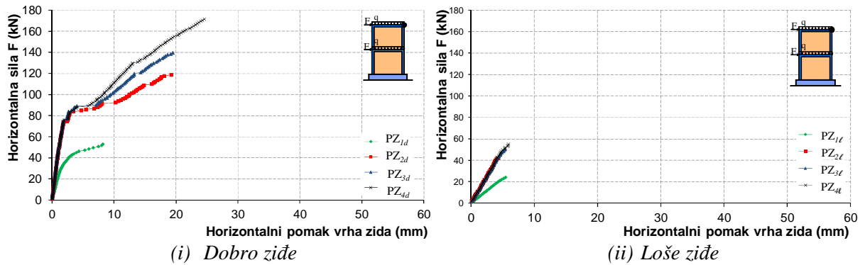
Slika 5.57. Horizontalni pomak vrha zidanih zidova bez otvora
