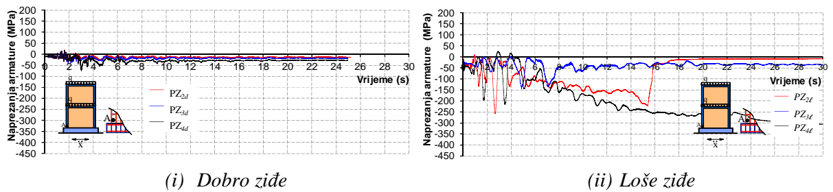
Slika 5.55. Utjecaj promjera vertikalnih šipki vertikalnih serklaža na naprezanje armature u točki A pri dnu serklaža zidanih zidova bez otvora
