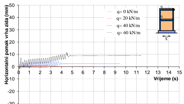
Slika 5.18. Horizontalni pomak vrha narmiranih zidanih zidova s otvorima
