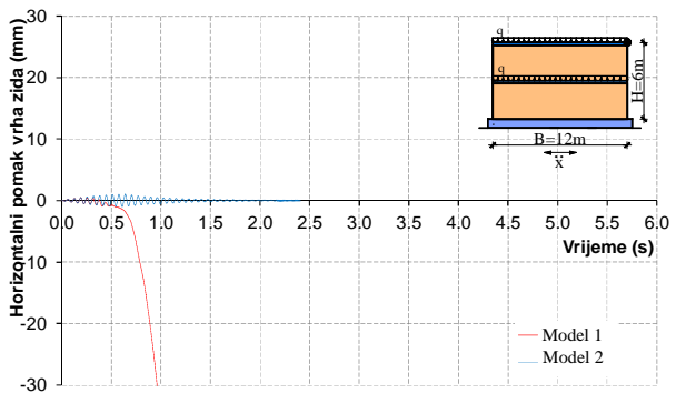
Slika 5.194. Horizontalni pomak vrha nearmiranih zidanih zidova izloženih harmonijskom ubrzanju podloge s a_{\max}=0,05g
