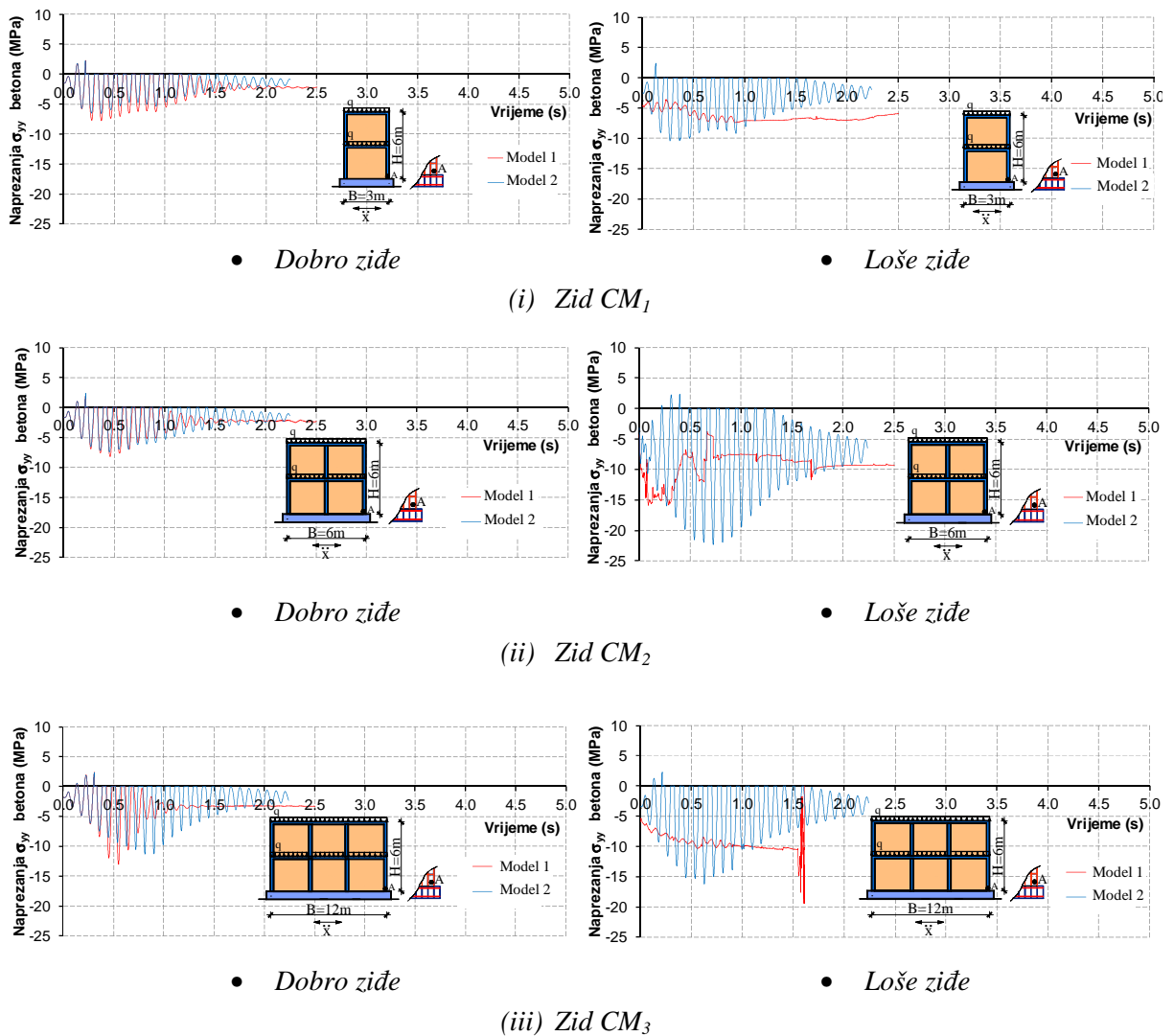
Slika 5.215. Vertikalno naprezanje u betonu u točki A omeđenih zidanih zidova izloženih harmonijskom ubrzanju podloge s a_{\max}=0,1g
