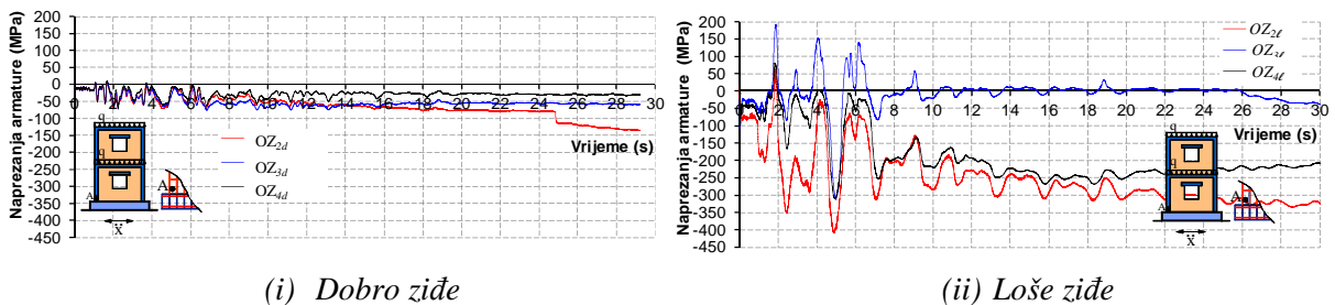
Slika 5.56. Utjecaj promjera vertikalnih šipki vertikalnih serklaža na naprezanje armature u točki A pri dnu serklaža zidanih zidova s otvorima
