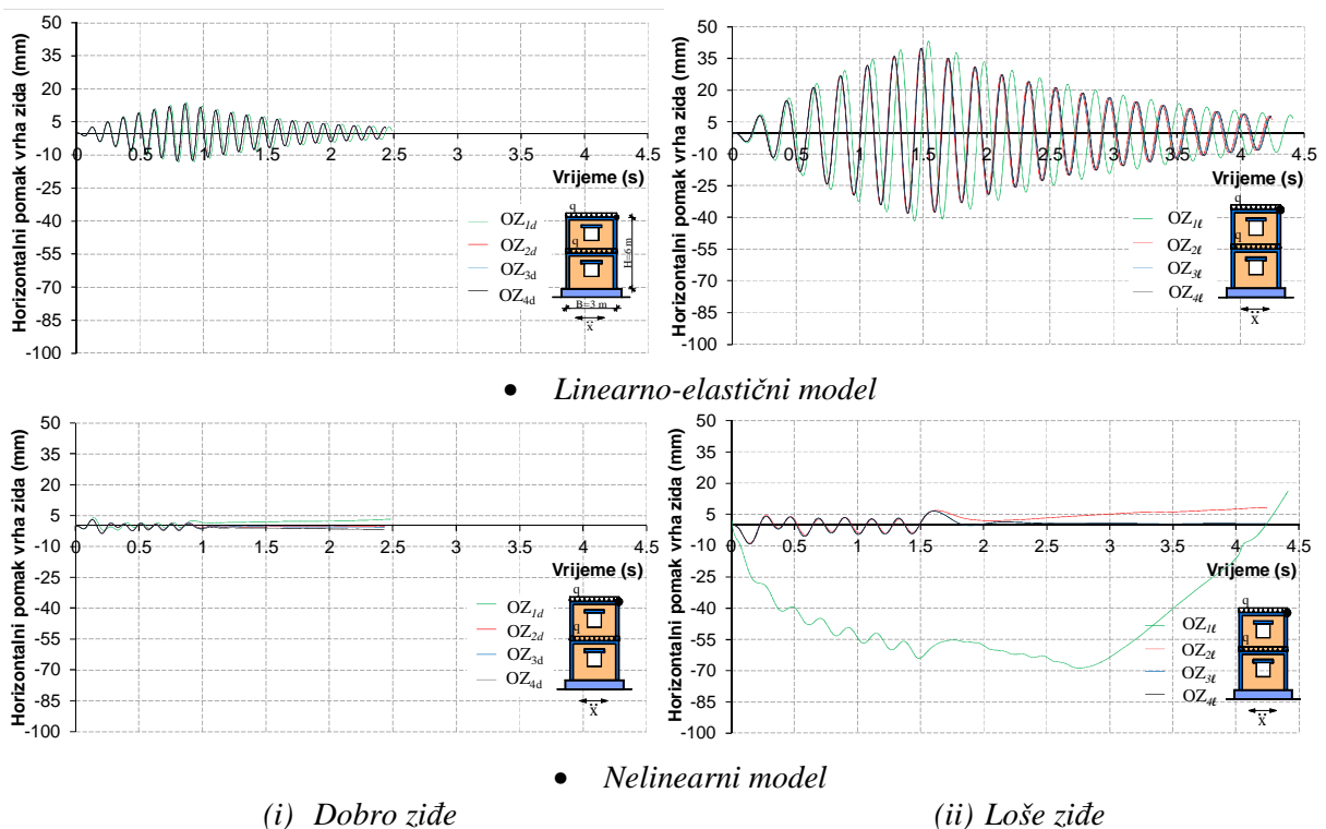
Slika 5.125. Horizontalni pomak vrha zidanih zidova s otvorima
